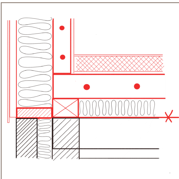
DETAIL GESCHOSSÜBERGANG
